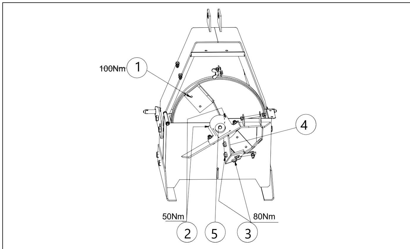
Bild 10. Checklista för åtdragning och kontroll av spel
