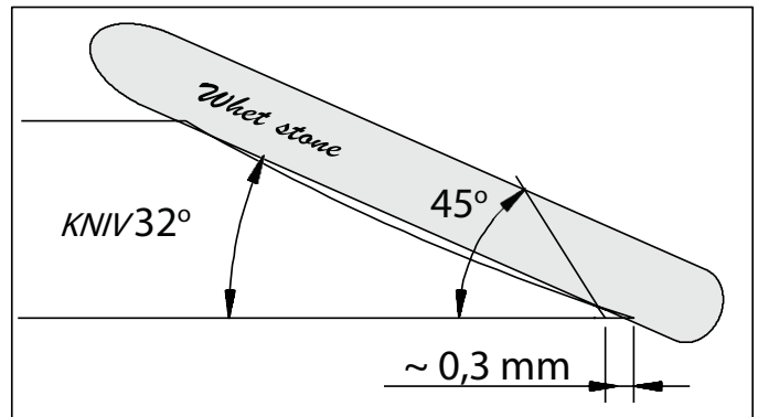
Bild 13. En konkav knivs profil
